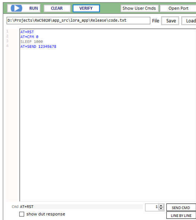
Fig 3.27 DUT Control
